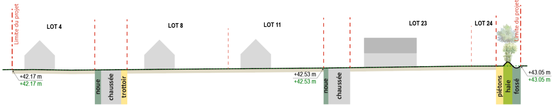
Coupe AA'
